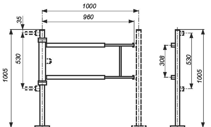
bramka dla personelu SW 026.000 SW 026.000 K – zamykana na klucz
